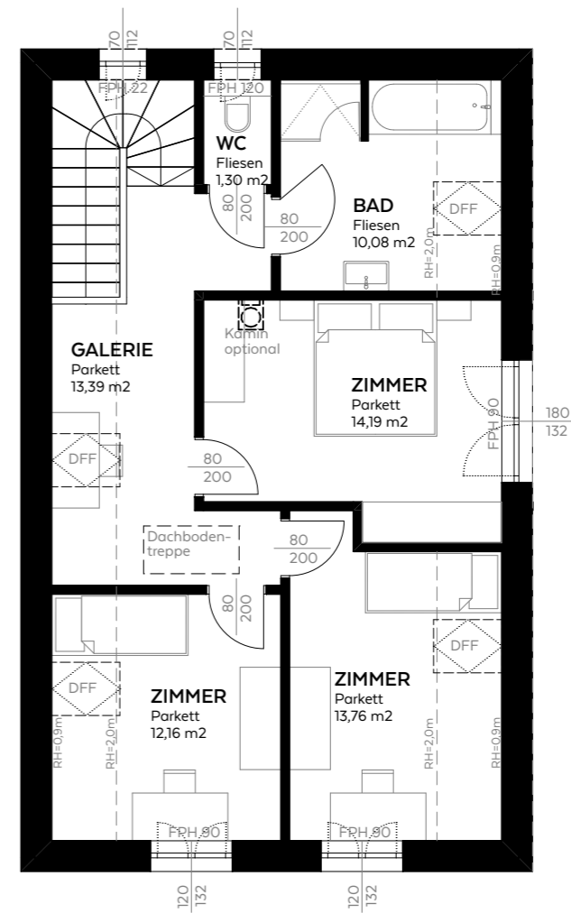
DACHGESCHOSS
