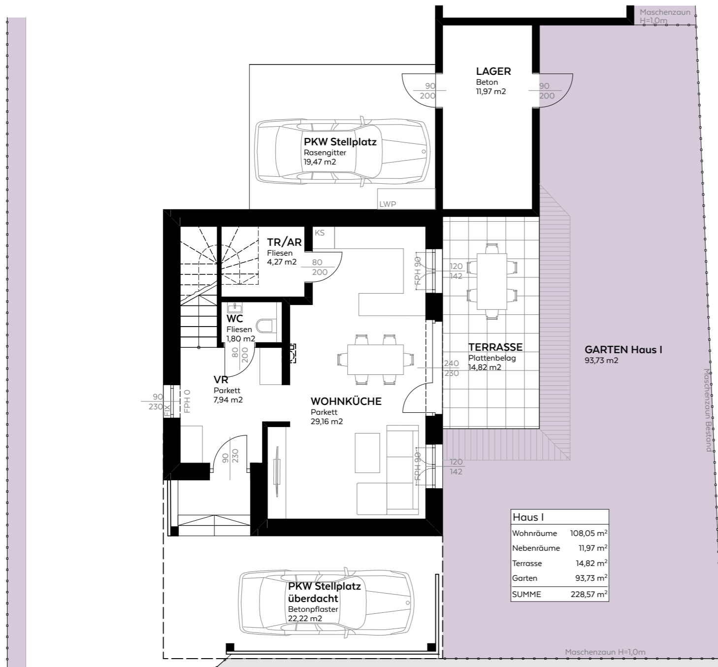
ERDGESCHOSS
